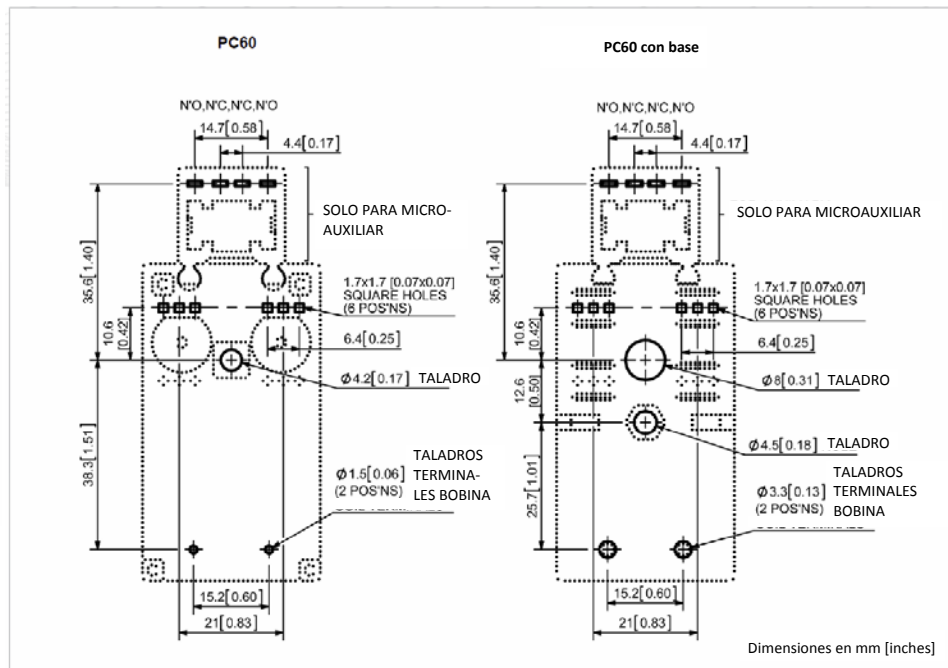
Contactor PC60 montado en base
