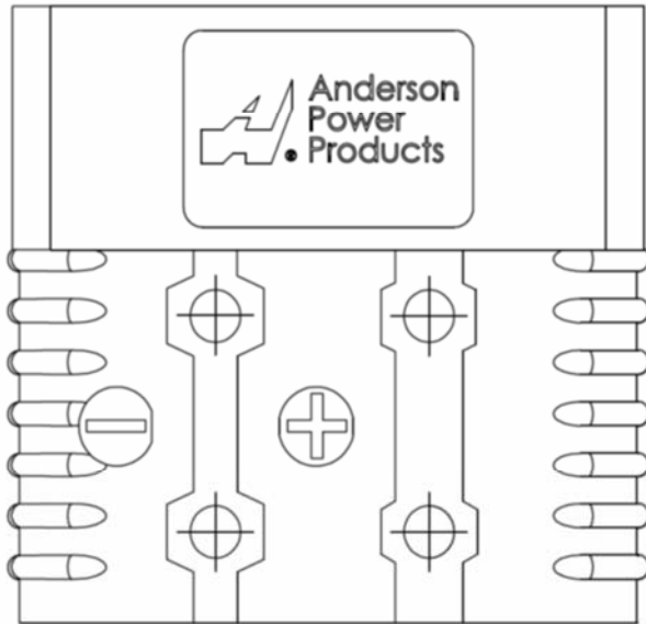
SB®175 - 3 Pole
